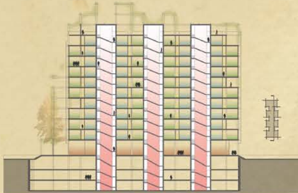
Schnitt BB
