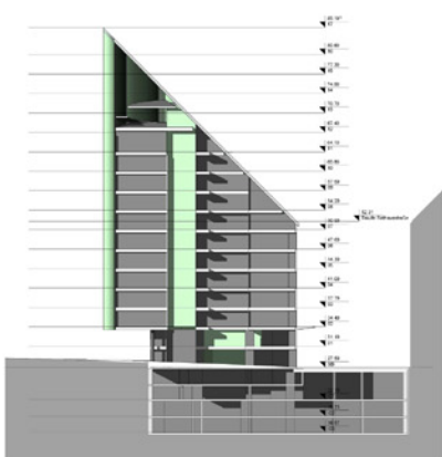
schnitt auerspergstraße - rathausstraße
