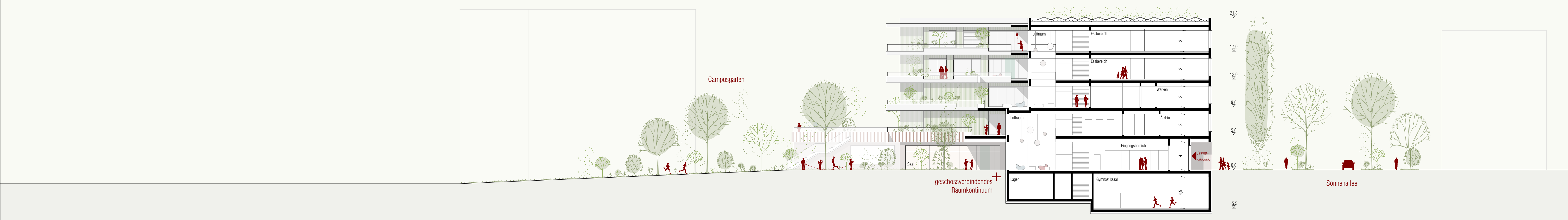
SNITT N-S EINGANGSBEREICH / MITTE . M 1:250
